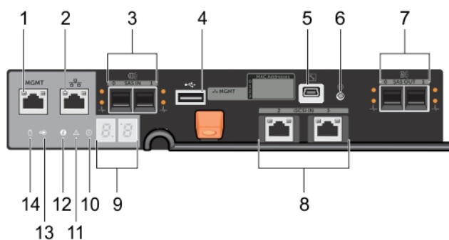
Figure 8. Voyants et fonctions du module de contrôleur RAID iSCSI MD3860i
